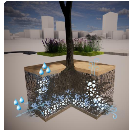
Prinzip des erweiterten Wurzelraumes
