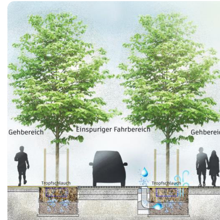
Straßenquerschnitt mit Entwässerung im Baumquartier
