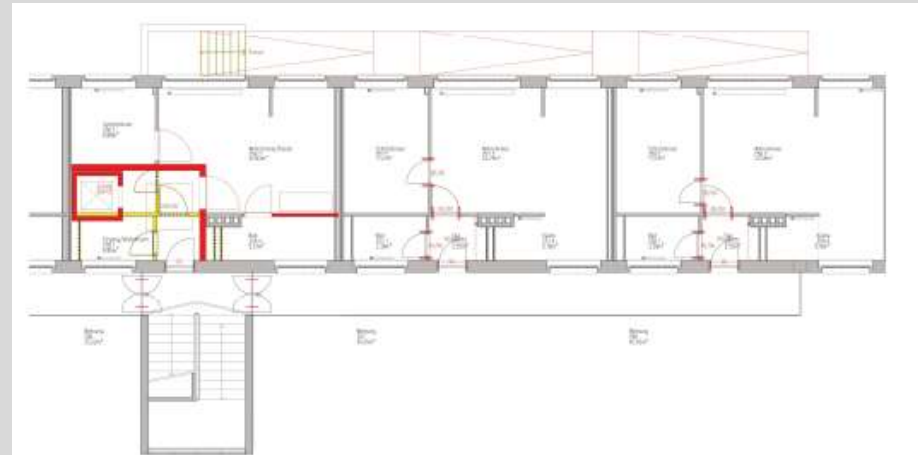
Konzept Aufzugeinbau / Grundriss Wohngeschosse, o.M.
