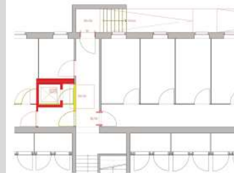
Konzept Aufzugeinbau / Grundriss-Ausschnitt Untergeschoss, o.M.
